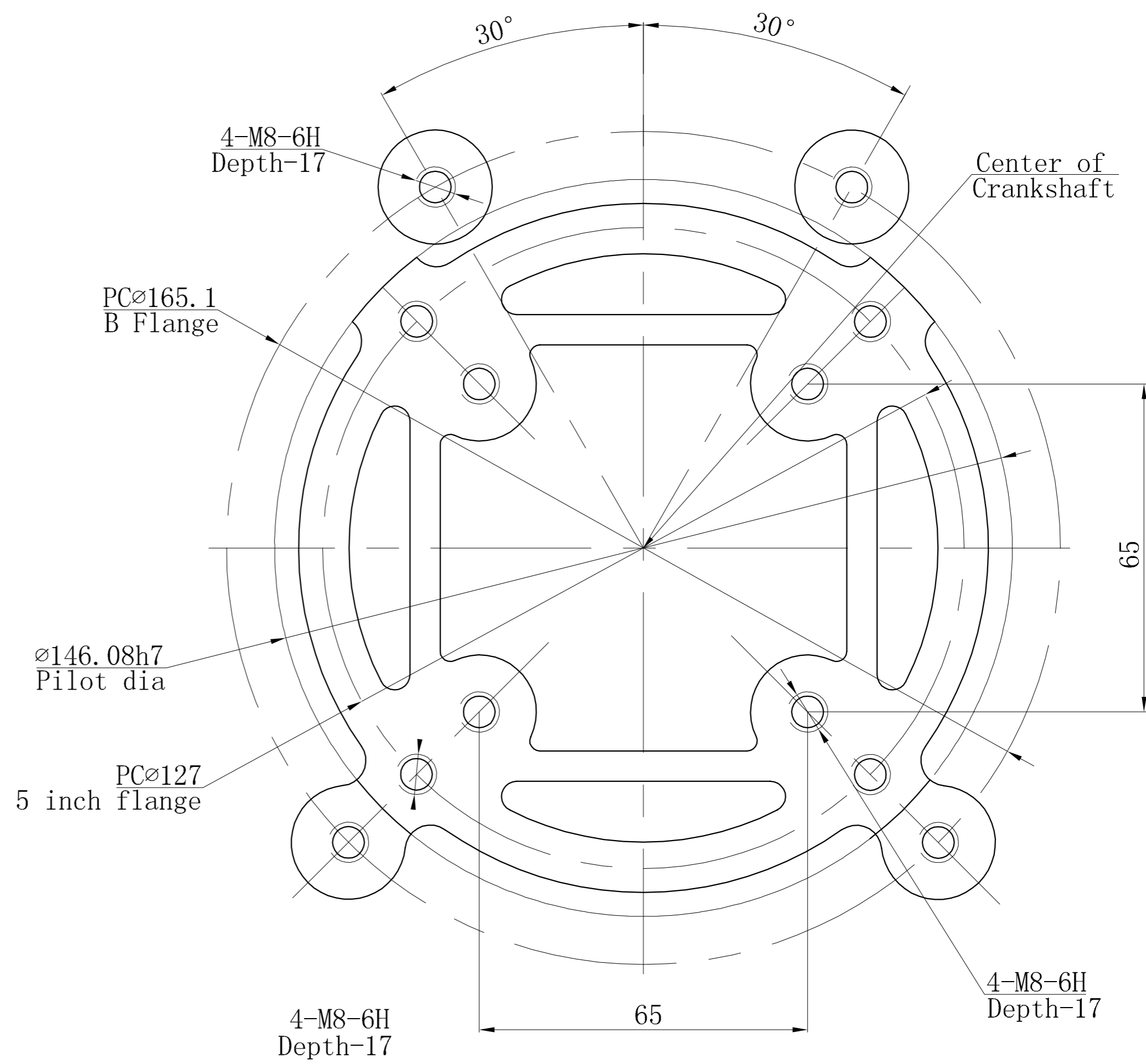
PTO Flange
