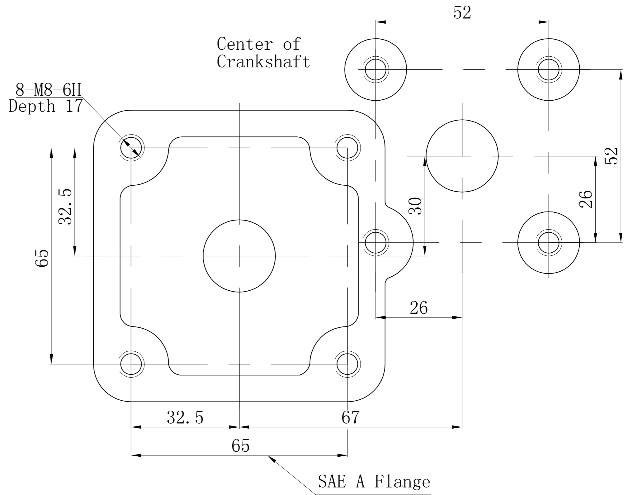
PTO Flange
